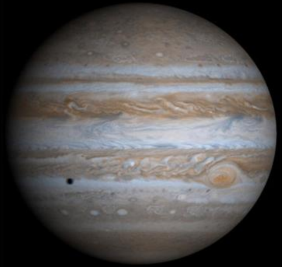
Bild der Raumsonde Cassini, NASA. Der Jupitermond Europa wirft seinen Schatten auf die Wolkenoberfläche des Planeten.
